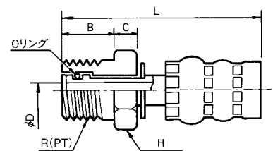
管用テーパおねじ (簡易スイベルタイプ)
