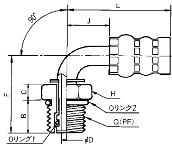
90°バンドフィッティング (平行ねじ簡易スイベルタイプ)
