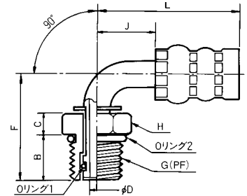
90°バンドフィッティング (平行ねじ簡易スイベルタイプ)
