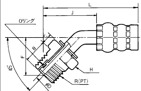
45°ベンドフィッティング (おねじ簡易スイベルタイプ)
