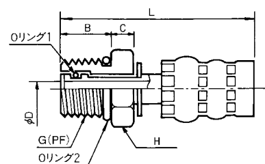
管用平行おねじ (簡易スイベルタイプ)
