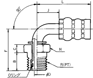
90°バンドフィッティング (おねじ簡易スイベルタイプ)
