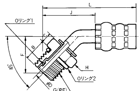
45°ベンドフィッティング (平行ねじ簡易スイベルタイプ)
