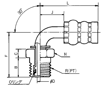
90°ベンドフィッティング (おねじ簡易スイベルタイプ)
