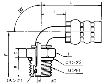
90°ベンドフィッティング (平行ねじ簡易スイベルタイプ)
