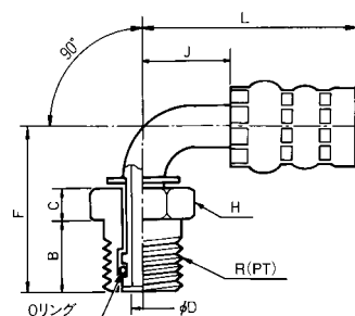
90°バンドフィッティング (おねじ簡易スイベルタイプ)
